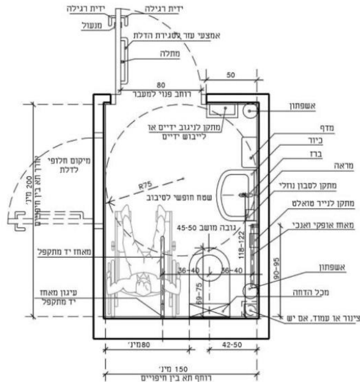
119א – תא בית שימוש נגיש מטיפוס 1, שיש בו אסלה עם מכל הדחה גלוי
