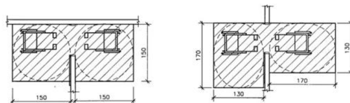
ציור 2 - משטחי תפקוד לפני דלת סובבת (המידות בסנטימטרים)
