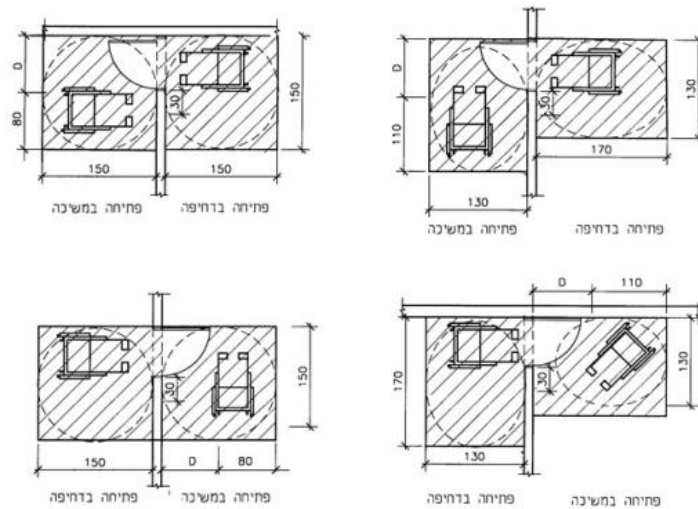
ציור 2 - משטחי תפקוד לפני דלת סובבת (המידות בסנטימטרים)
