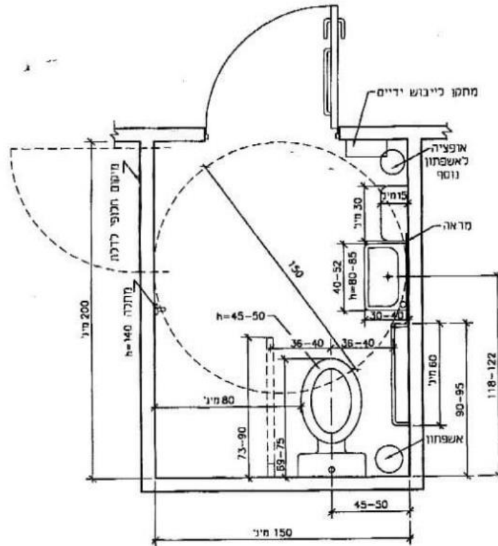
צויר 16 - תא שירותים עם אסלה פינתית (המידות בסנטימטרים)
